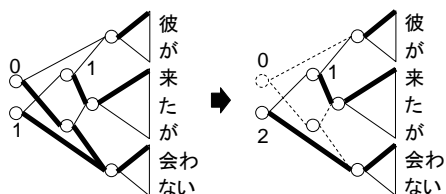
図 3: 統語森係り受け解析による最尤構造推定
