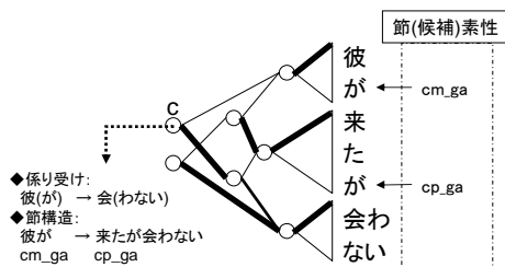
図 2: 節点における尤度計算
