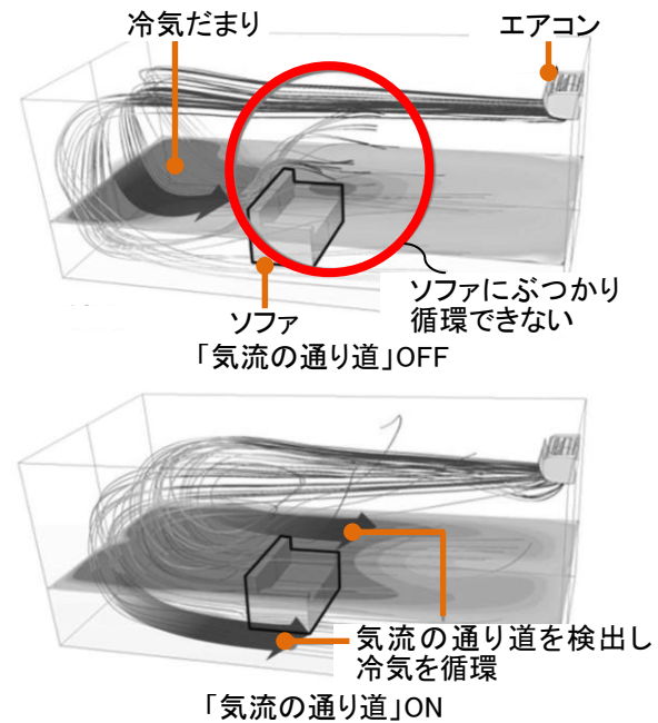
図5 冷房運転時の「気流の通り道」
