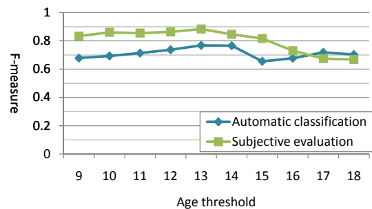
図9 子ども判別のF値による比較
