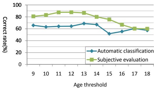
図7 子ども判別における正解率の比較
