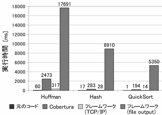
図 10 実行時間
