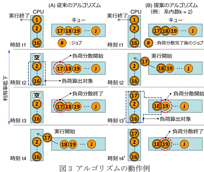
図3 アルゴリズムの動作例
